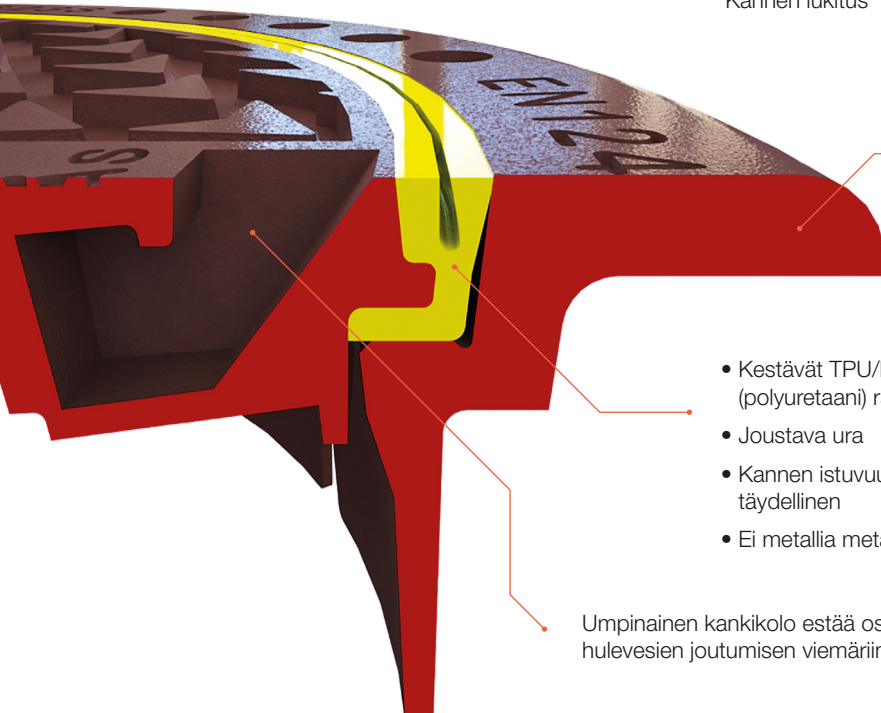
Kannen lukitus
